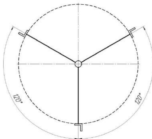
Рисунок 1 – Схема размещения растяжек в плане
